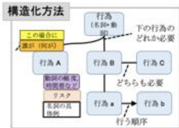
図 1: 可読性を向上した CHARM による知識表現形式の凡例。
