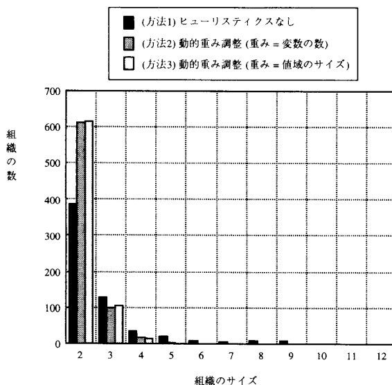
図3 組織形成のようす ( n=30 の場合)
