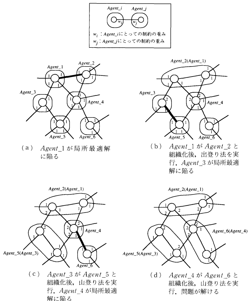
図2 動的重み調整
