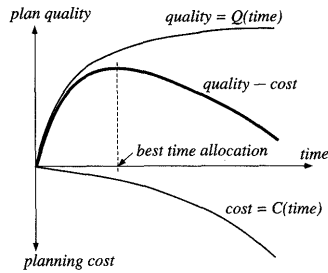
図8 情報処理の価値とコストのトレードオフ。関数 Q が性能曲線である。この図は [Horvitz 87] に基づいている
