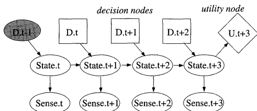
図 4 動的決定ネット [Forbes 95]. 正方形は決定ノード、菱形は効用ノードを表す。
