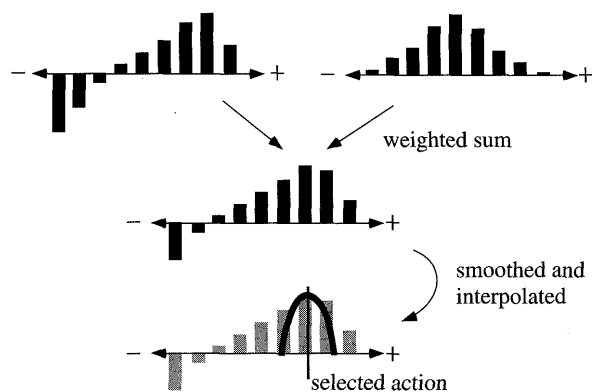
図6 DAMNにおけるコマンドレベルの統合. この例では、二つの判断器が各行動候補(横軸)について適切度を計算し、それらの重み付け和として適切度を統合している。[Rosenblatt 97]の図を一部改変
