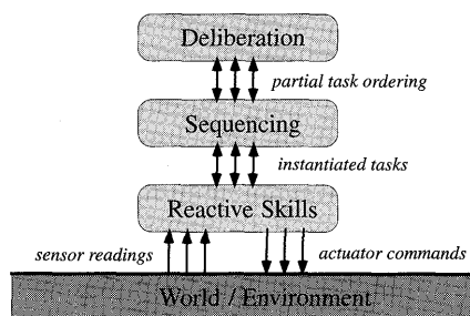
図7 3Tアーキテクチャ[Bonasso 97]
