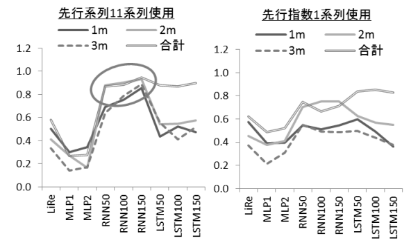
図 17: 相関係数(テストデータ 5)
